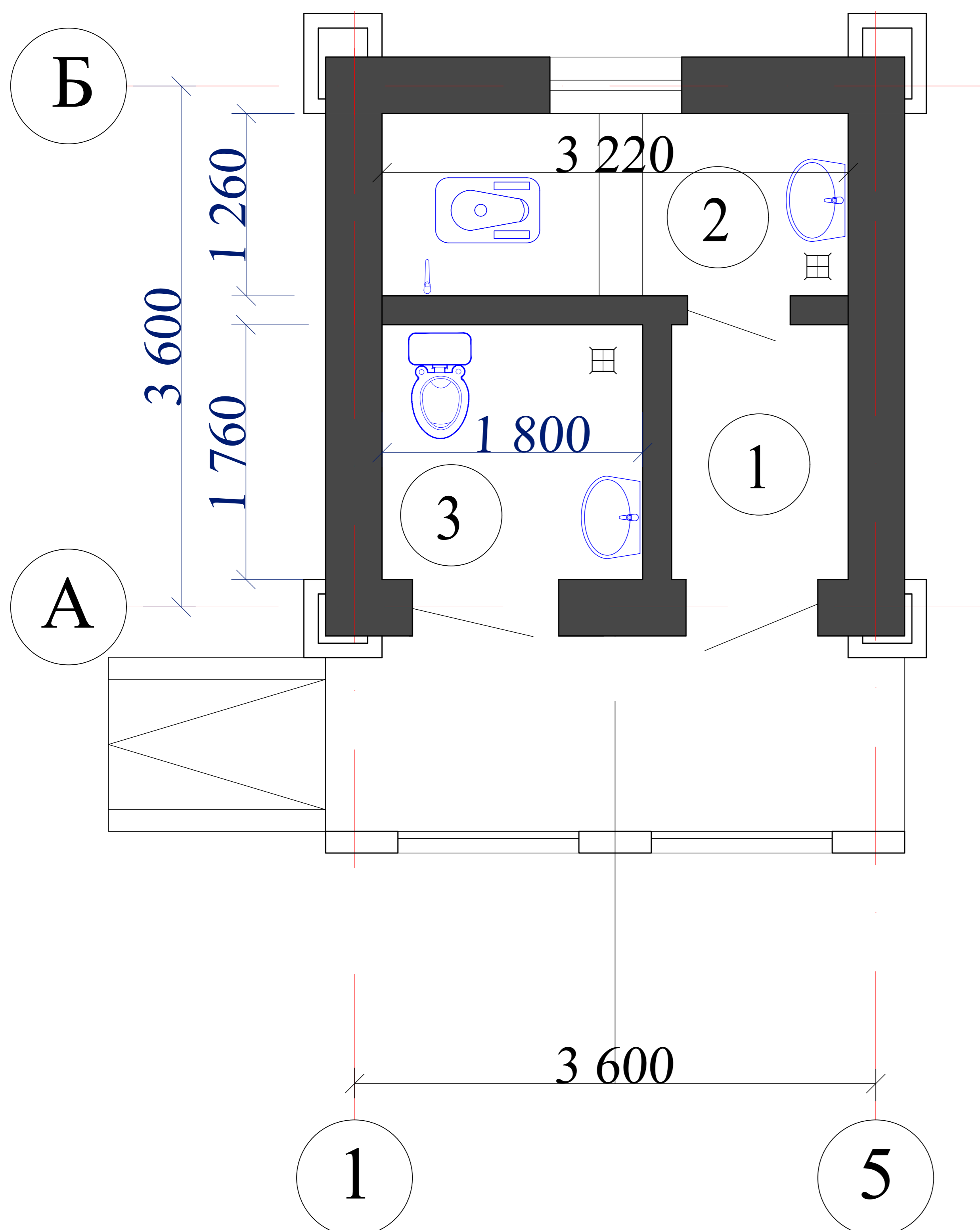
План стен
